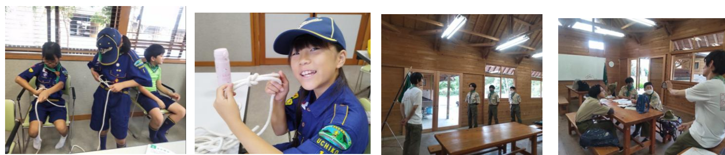
もやい結び
