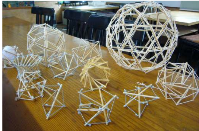
テンセグリティーの見本
